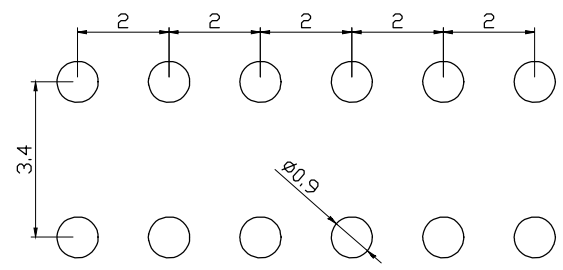
安装图 (PCB LAYOUT PLAN)
