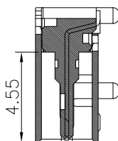
剖面图 A-A
