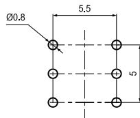
印制线路板 Recommended P.C.B layout
