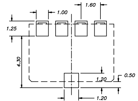
推荐PCB版布局
