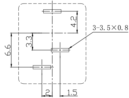
线路板开孔尺寸 TOP VIEW
