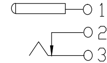
电路原理图
