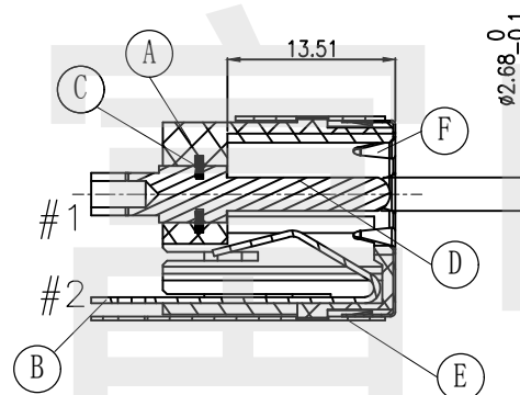
A-A' SECTION
