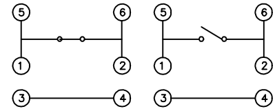
常态通电 按下 不通电 电路图
