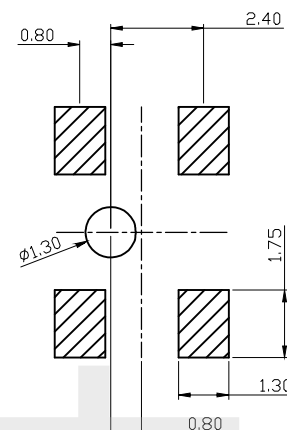
安装参考图
