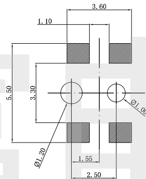
PCB. 焊接尺寸图
