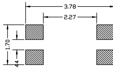
PCB. 焊接图
