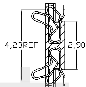
剖面 A-A
