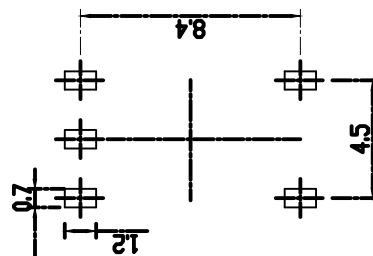
PCB. 焊接图
