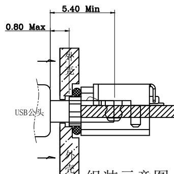
组装示意图
