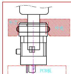
组装示意图
