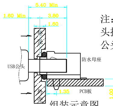
组装示意图
