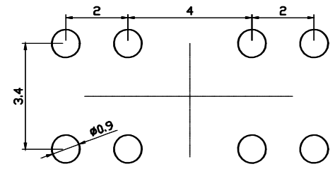
安装图 (PCB LAYOUT PLAN)
