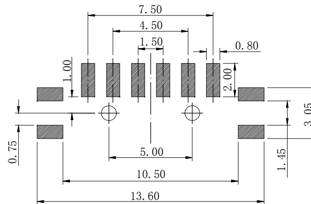
PCB 焊接尺寸图
