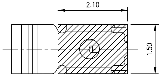
焊盘尺寸 尺寸公差 ±0.05
