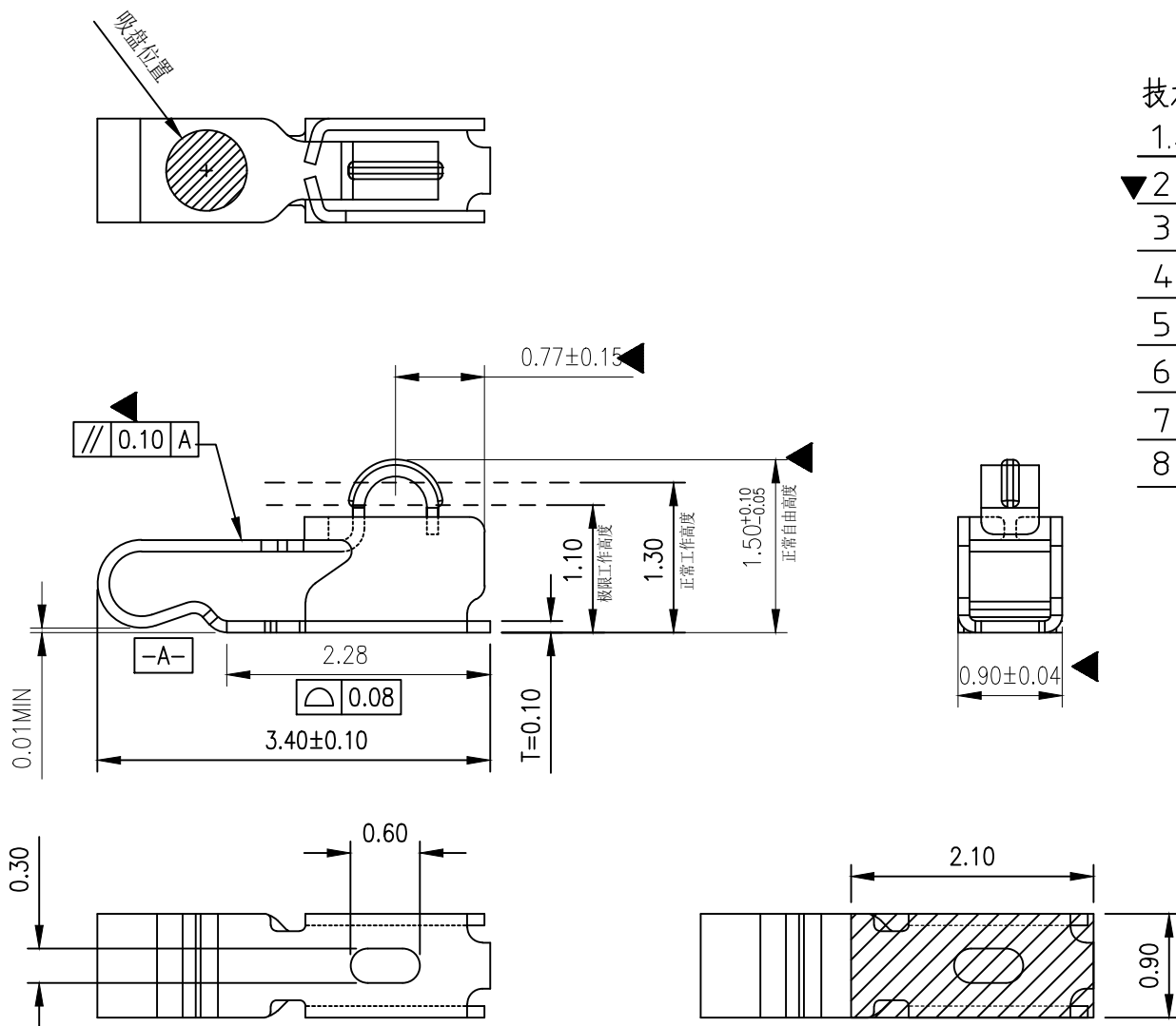
焊盘尺寸 尺寸公差 ±0.05
