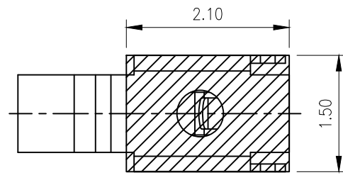
焊盘尺寸 尺寸公差 ±0.05
