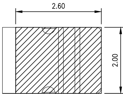
焊盘尺寸
