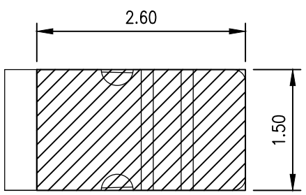
焊盘尺寸 尺寸公差 ±0.05
