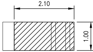
焊盘尺寸 尺寸公差 ±0.05
