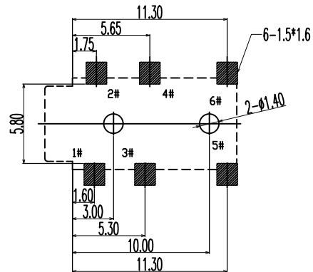
P.C.B LAYOU TOP VIEW
