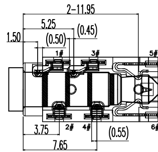
5 极插头接触点位置尺寸
