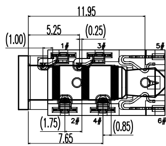
4 极插头接触点位置尺寸
