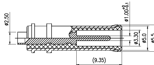
DC-MATEING PLUG<REF>
