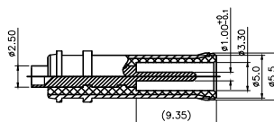
DC-MATEING PLUG(REF)
