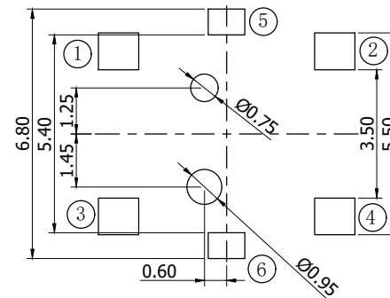
P.C.B SOLDER LAND DIMENSION
