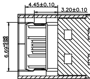
截面:A-A
